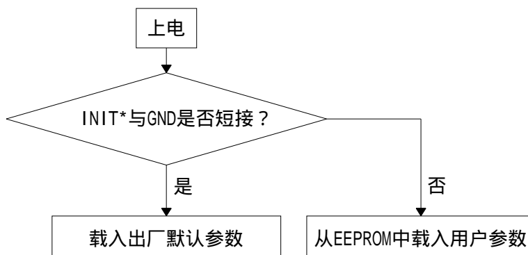
图2.3 IR-2031 启动过程及参数载入流程图
