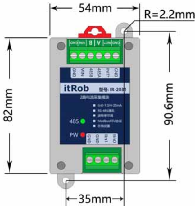
图1.3 IR-2031尺寸
