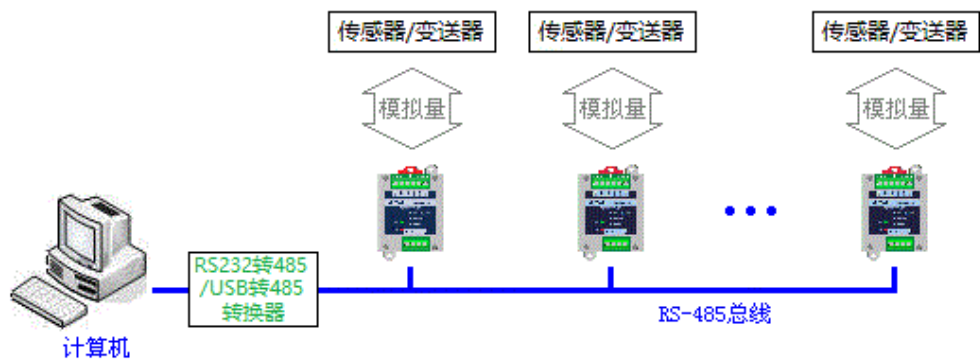
图2.1 IR-2031典型应用
