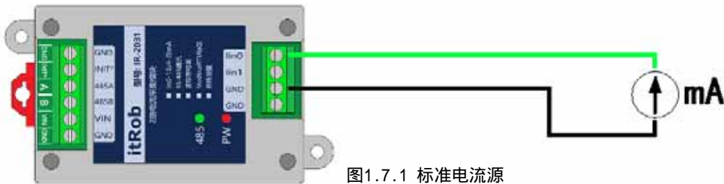
图1.7.1 标准电流源
