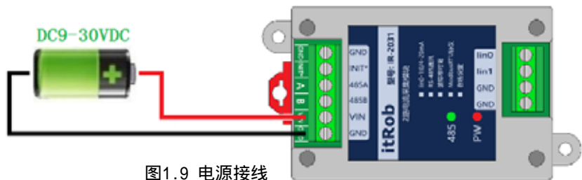
图1.9 电源接线
