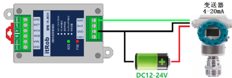
图1.7.3 三线制接线示意图
