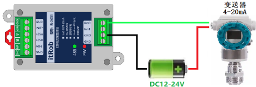
图1.7.2 与两线制变送器接线示意图
